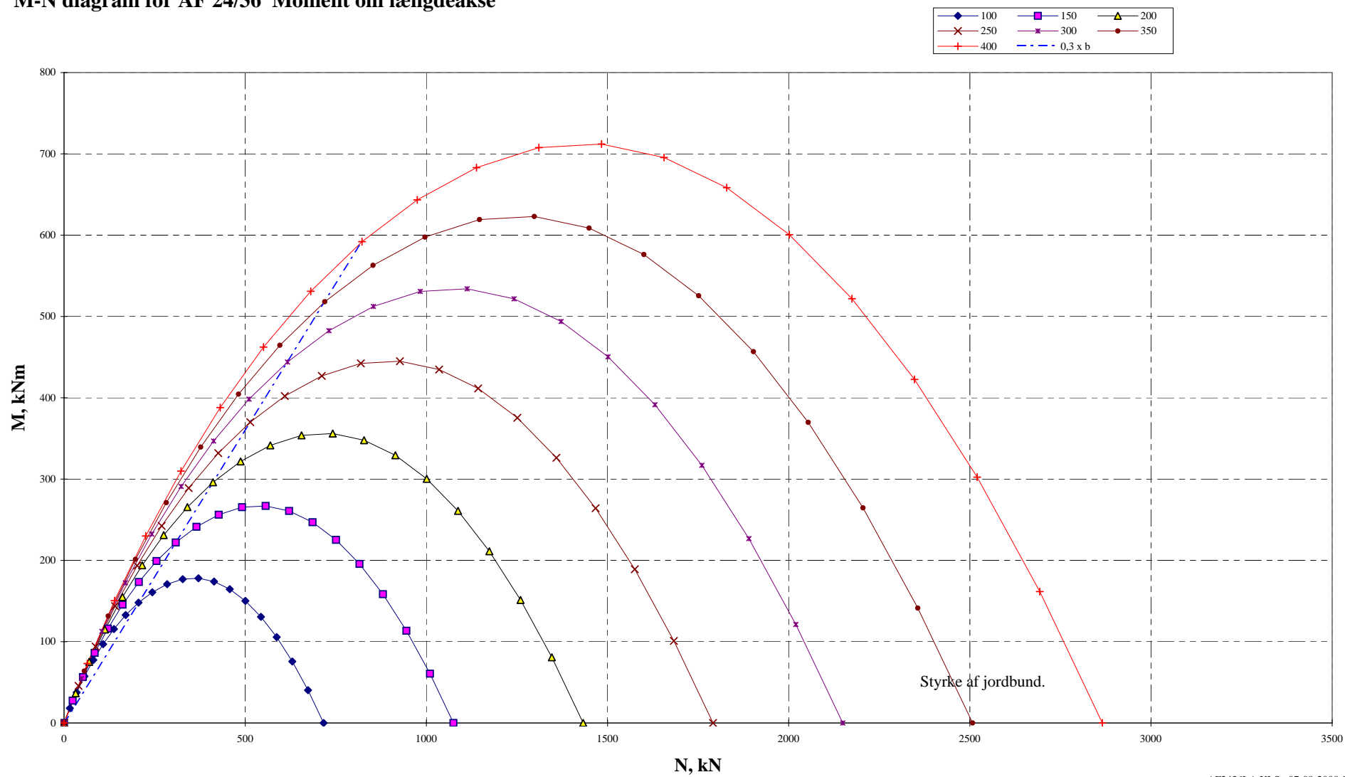
M-N diagram for AF 24/36 Moment om længdeakse
