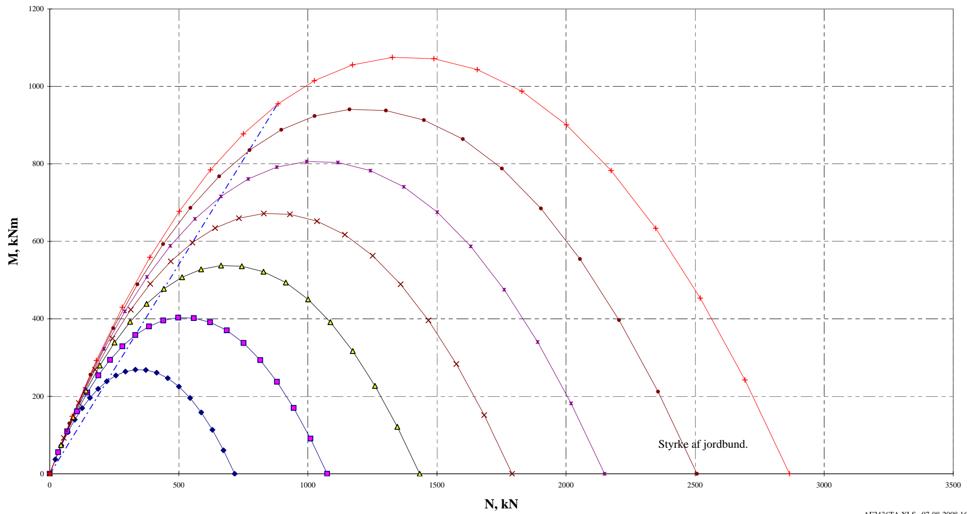
M-N diagram for AF 24/36 Moment om tværsakse
